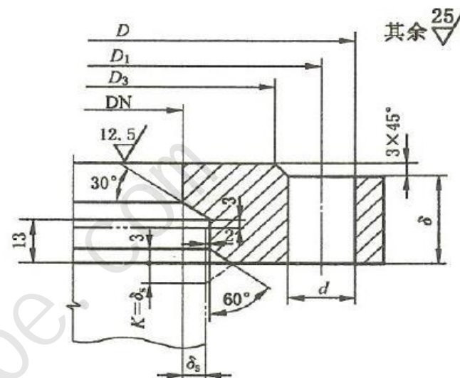
图 10-1 平密封面法兰
